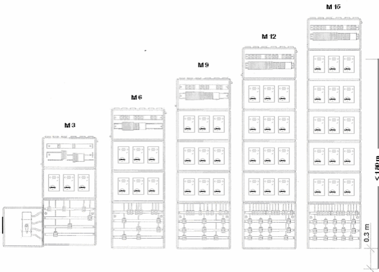
Fig. 3 : Ejemplo de cuadro modular tipo A de tres huecos (con envoltente)
