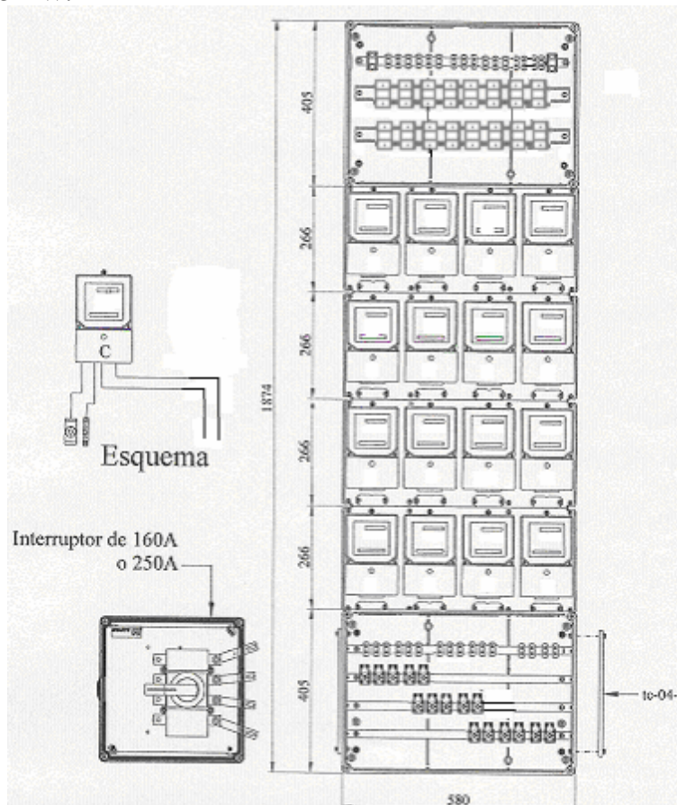
Fig. 12 a: Cuadro modular tipo A de cuatro huecos (sin envoltente)
