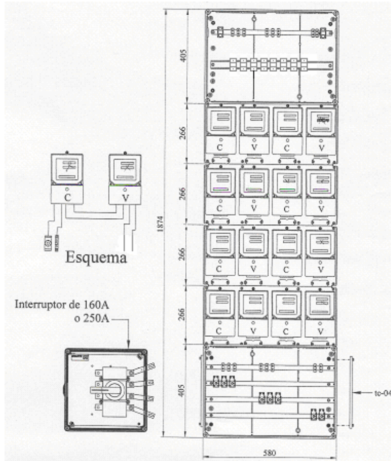
Fig. 12: Cuadro modular tipo A de cuatro huecos (sin envolvente)
