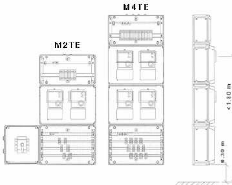
Fig. 14: Cuadro modular tipo E M (con envolvente)
