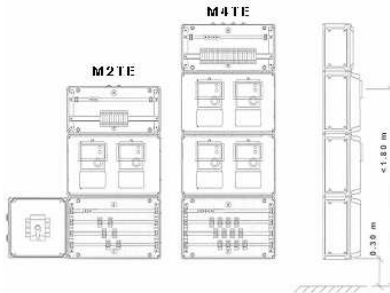
Fig. 11: Cuadro modular tipo E M (con envolvente)
