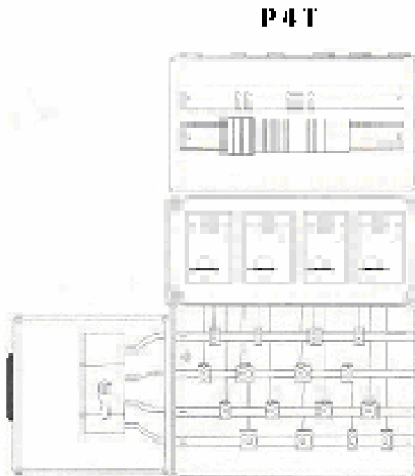
Fig. 8: Cuadro modular tipo A de 4 huecos (sin envoltente)
