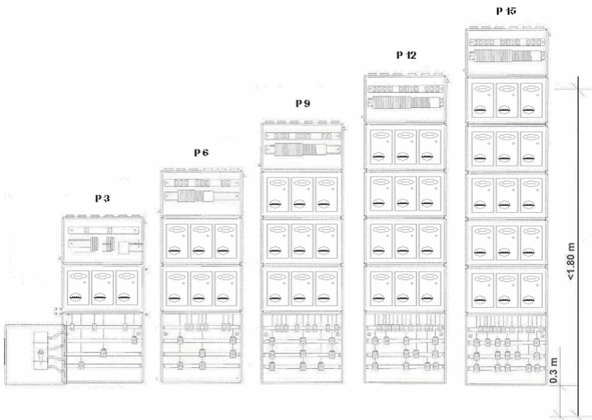
Fig. 2 : Ejemplo de cuadro modular tipo A de tres huecos (sin envolvente)
