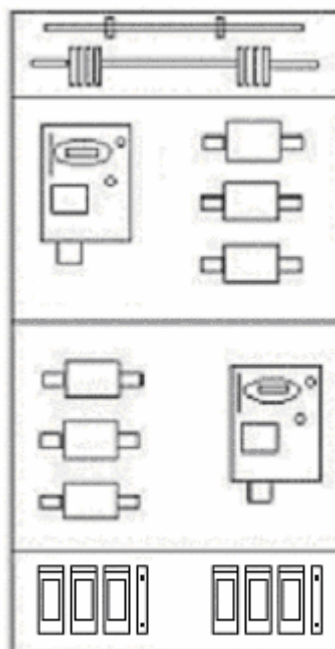
Fig. 15: Ejemplo de cuadro modular tipo A para 1 ó 2 equipos de medida de 63 / 120 A.
